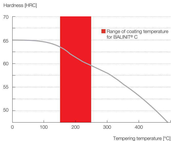
Tempering diagram for AISI 52100 / DIN 1.3505
